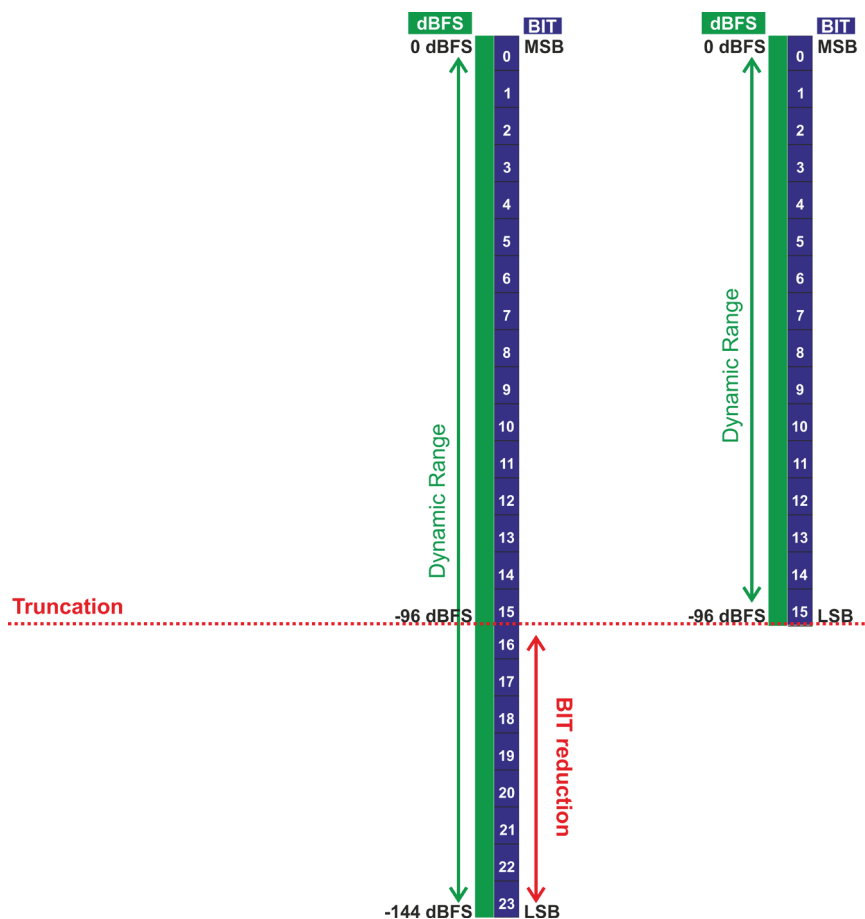
fig. 13.2 Troncamento da 24 a 16 Bit
