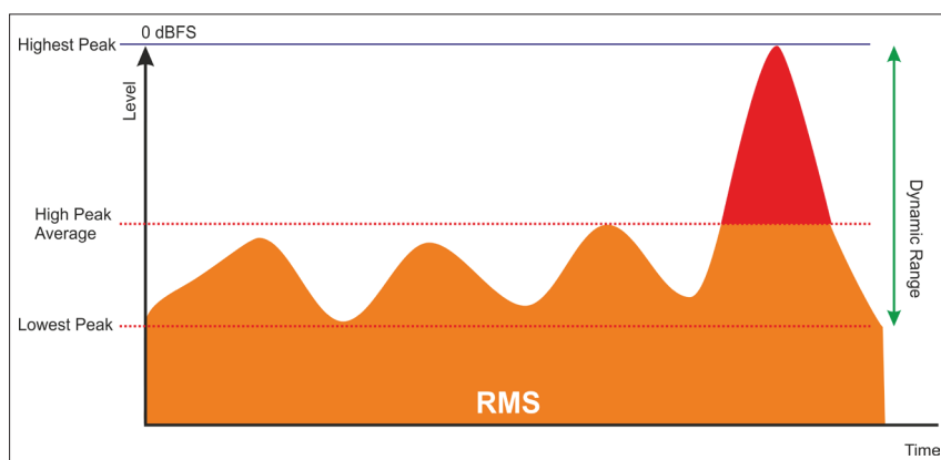
fig.7.2 Segnale non compresso
