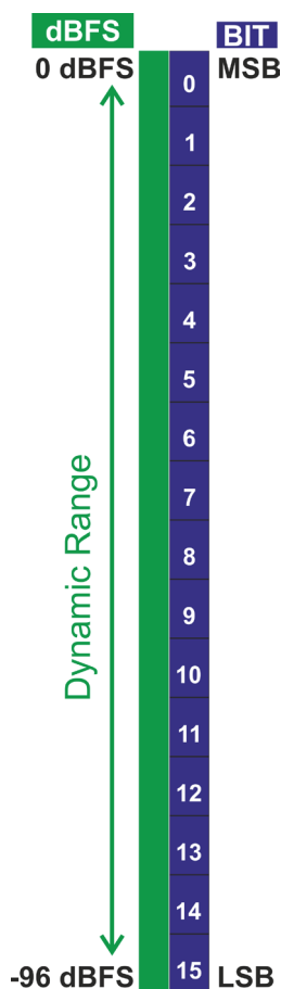
fig. 13.1 Rapporto tra bit e range dinamico
