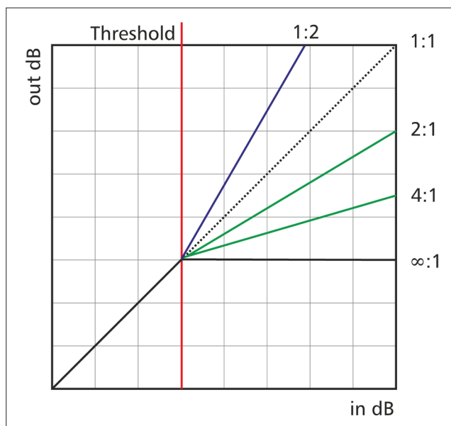
fig. 7.1 Rappresentazione grafica della funzione di un processore dinamico
