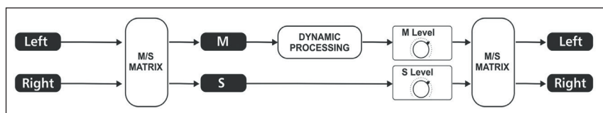
fig. 10.1 Processamento dinamico M/S
