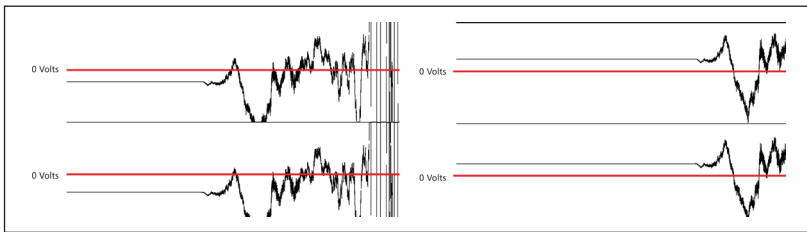
fig. 5.2 Errore di eliminazione di DC offset tramite tensione inversa
