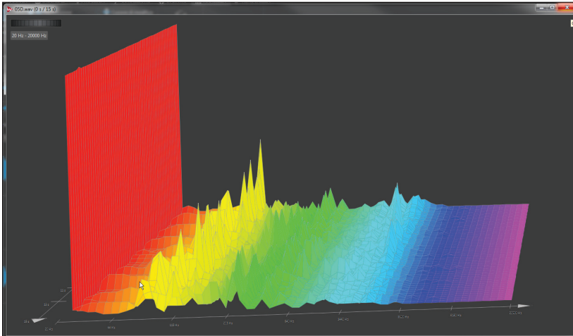
fig. 5.11 Analisi FFT di DC offset
