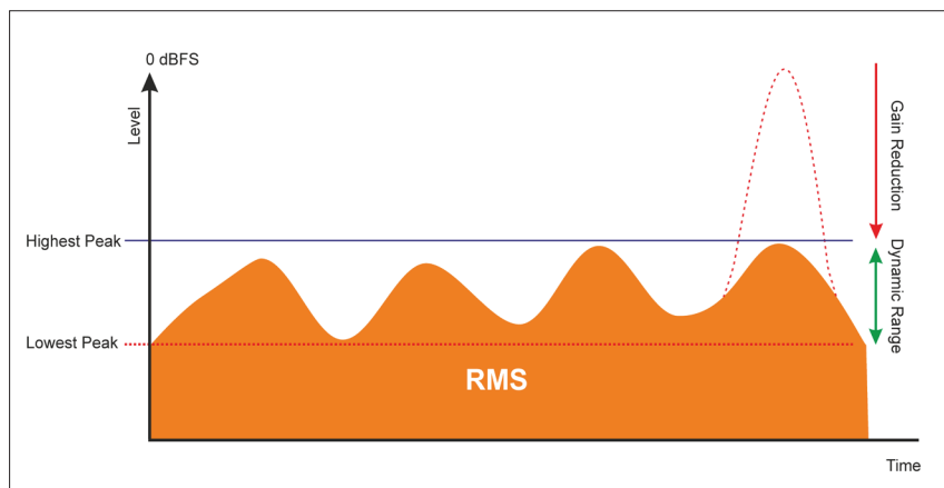
fig. 7.3 Segnale compresso
